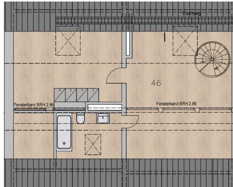
Spitzboden
