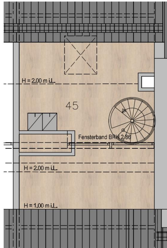
Spitzboden
